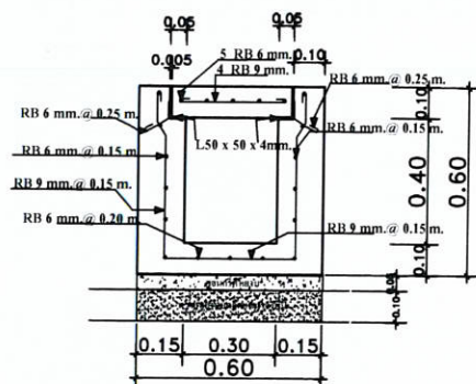
ภาพตัดแสดงรายละเอียดเหล็กเสริมราง คสล.
