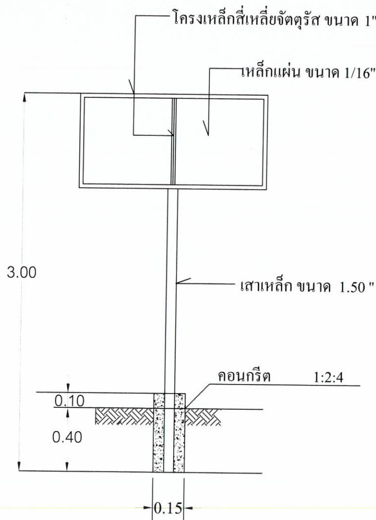
รูปตัด
