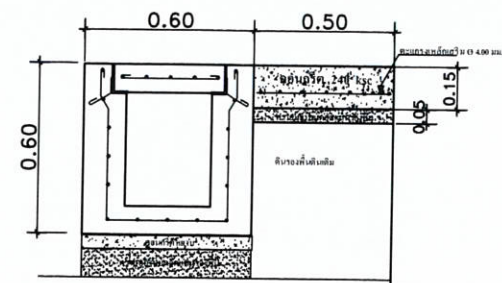
ภาพตัดแสดงรายละเอียด ผิวทาง คสล.
