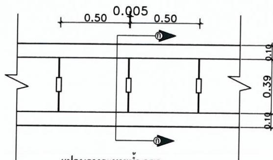
แปลนรางระบายน้ำ คสล.
