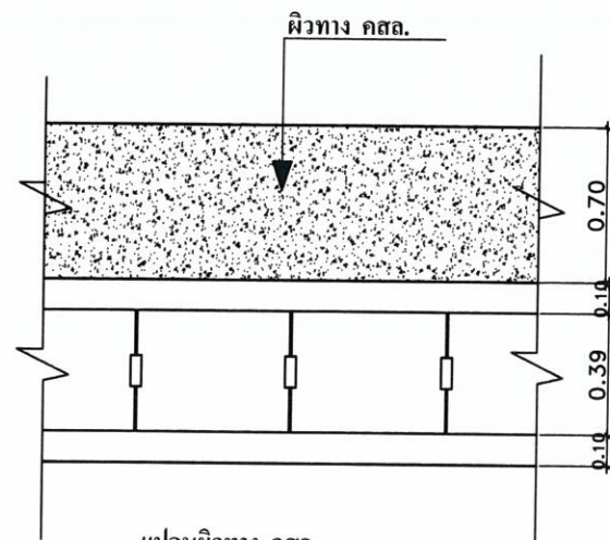
แปลนผิวทาง คสล.
