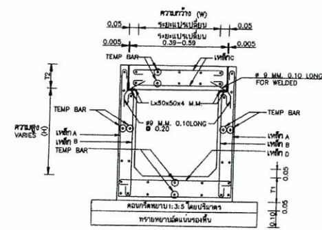
รายละเอียดหลักเสริมรางวัล คสช
