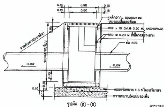
รูปตัด ๕ - ๕
