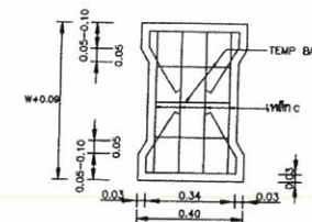
รายละเอียดหลักเสริมฟาราง คสล.
