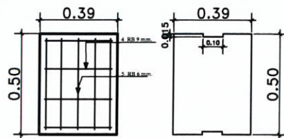
รายละเอียดเหล็กเสริมฝาราง คสล.
