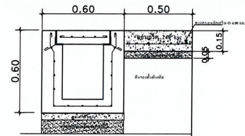
ภาพตัดแสดงรายละเอียด ผิวทาง คสล.
