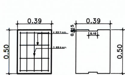
รายละเอียดเหล็กเสริมฝาราง คสล.
